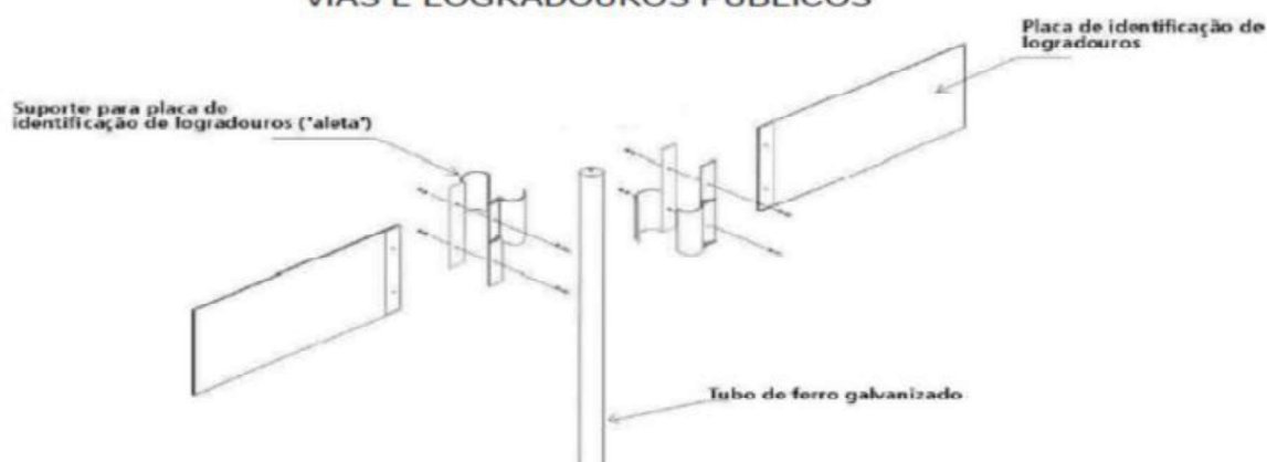
Figura 01: Perspectiva esquemática da fixação de placas de logradouro.
