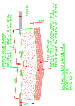
DETALHE DO SARJETÃO (CORTE-AA) ESCALA 1:100
