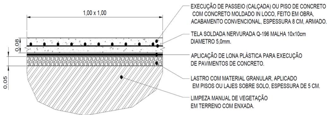
DETALHE EXECUTIVO DA CALÇADA
